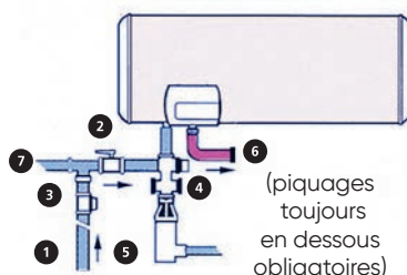
Horizontaux Muraux raccordement dessous
