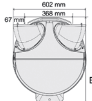
Bouche orientée vers l'arrière
