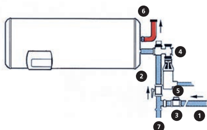
Horizontaux Muraux raccordement côté
