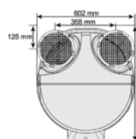
Bouche orientée vers le haut
