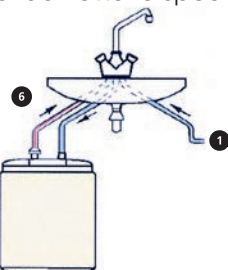
Écoulement libre avec robinetterie spéciale
