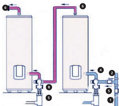
Montage en série 1
