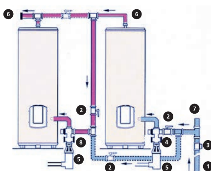
Montage en série parallèle 1
