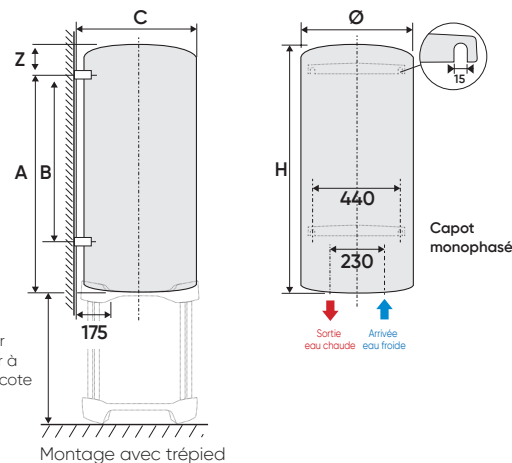
Montage avec trépied
