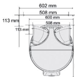
Bouche orientée vers le côté
