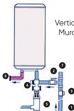
Montage en série parallèle 1
