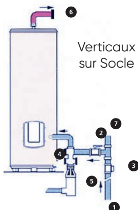
Montage en série 1
