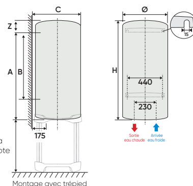
Montage avec trépied
