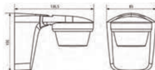
Plan d'encombrement
