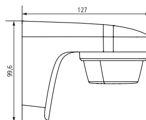
Plan d'encombrement
